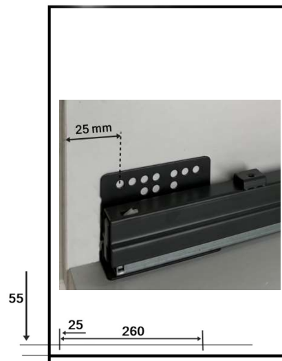
Lateral izquierdo
